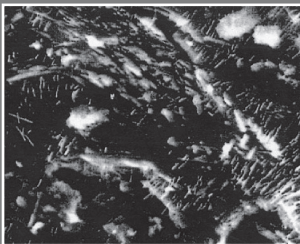
CALCESTRUZZO TRATTATO CON XYPEX
